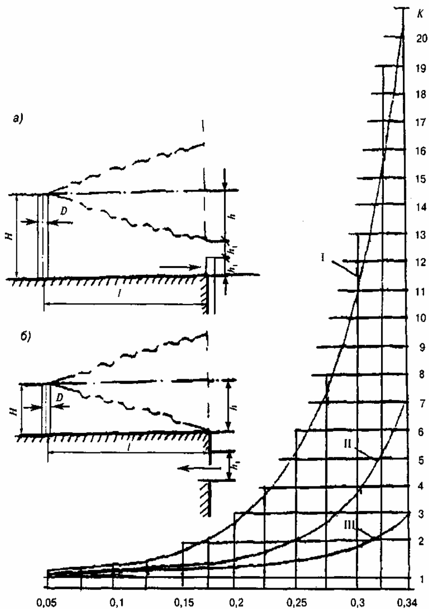
а - расположение источника над зоной всасывания наружного воздуха приемным устройством (высота трубы источника H=2h_1+h ); б- то же, над кровлей здания (высота трубы источника H=h ); h - расстояние по вертикали, м, горизонтальной оси струи; h_1 , - высота отверстия для приема наружного воздуха, м; l - расстояние между устьем источника и приемным устройством для наружного воздуха, м.
